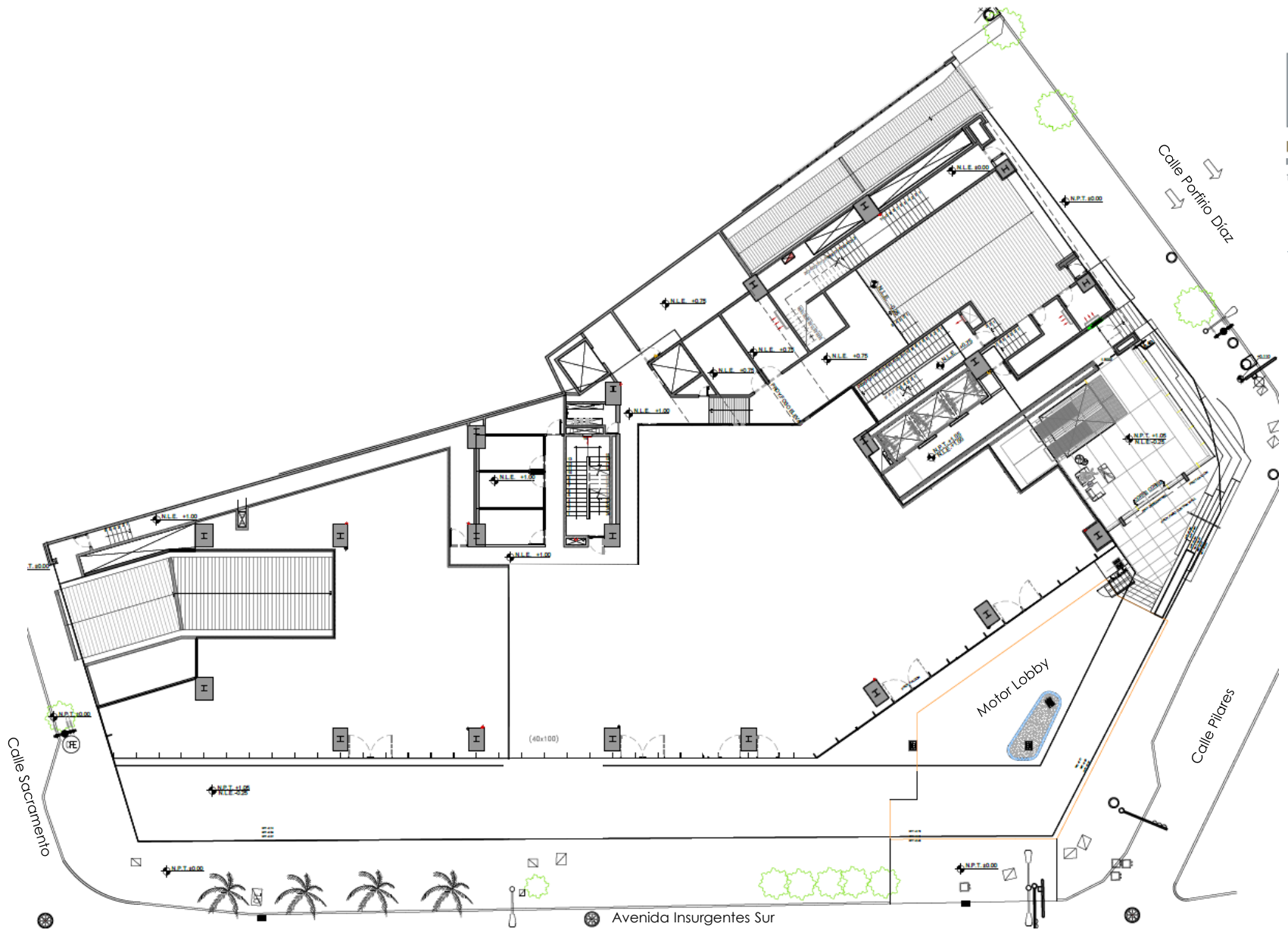
Planta Baja
